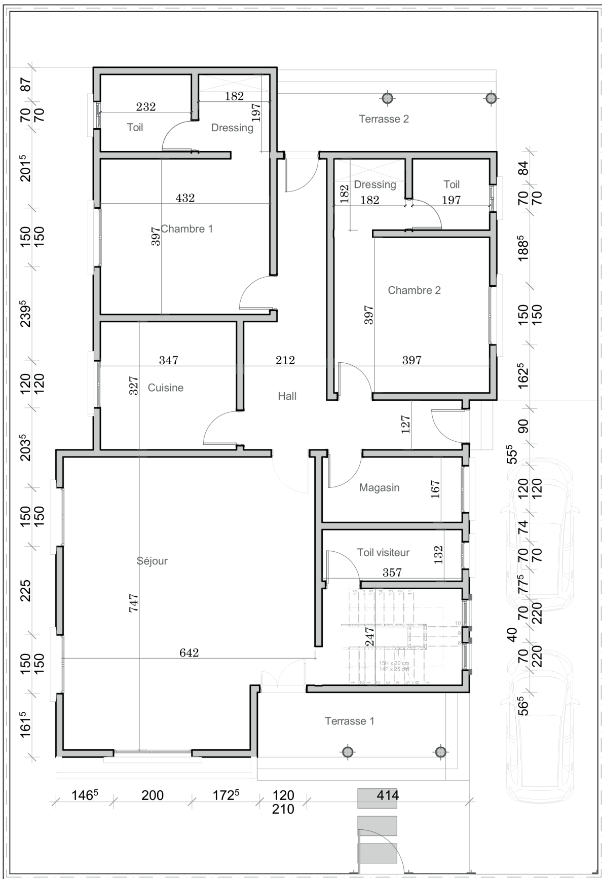
PLAN TYPE RDC
